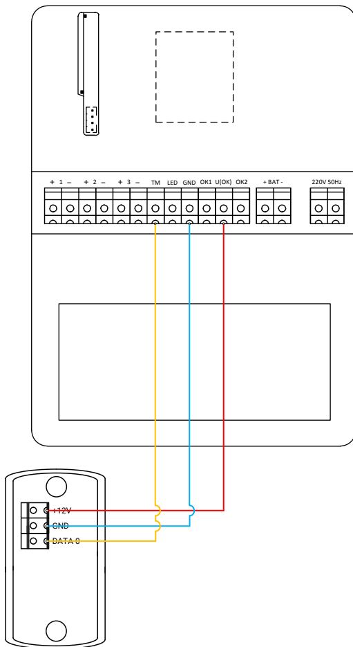
Рисунок 13. Схема подключения считывателя «Matrix-II»
