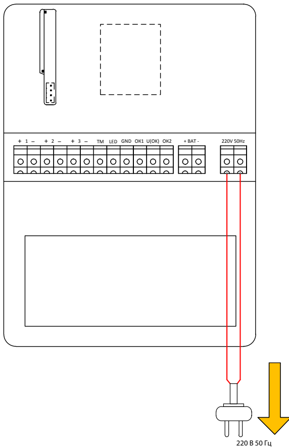
Рисунок 1. Схема подключения к сети 220В
