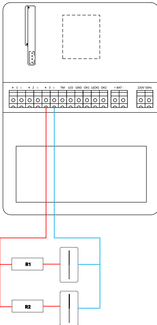
Рисунок 5. Схема подключения резистивных охранных шлейфов
