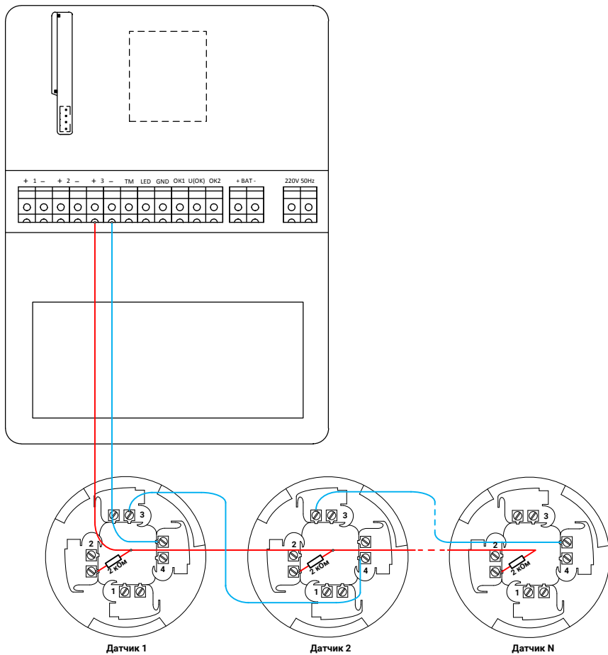
Рисунок 6. Схема подключения пожарных шлейфов
