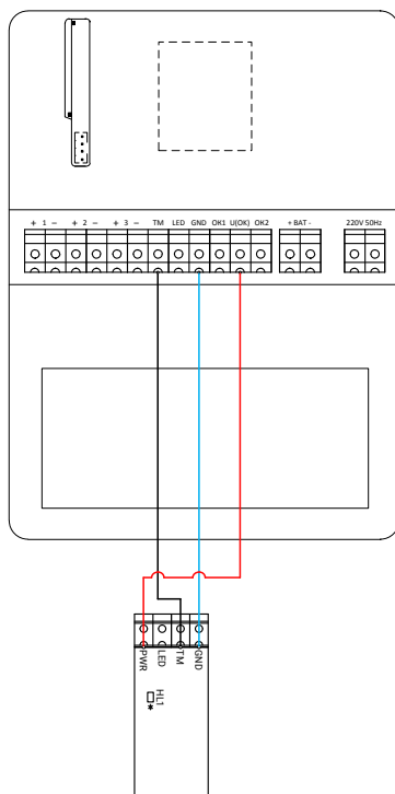
Рисунок 12. Схема подключения считывателя «MIF2-1»
