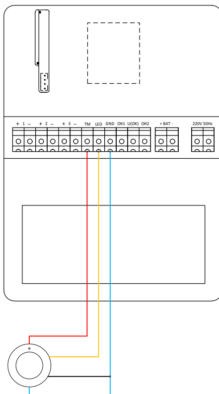
Рисунок 11. Схема подключения считывателя ТМ
