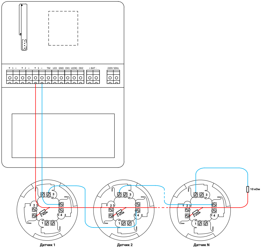
Рисунок 9. Схема подключения пожарных шлейфов с контролем обрыва
