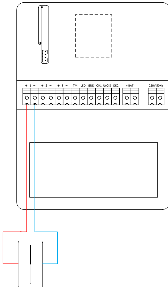
Рисунок 4. Схема подключения охранных шлейфов типа «сухой контакт»
