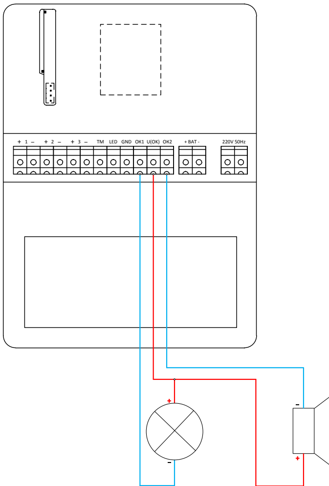
Рисунок 15. Схема подключения исполнительных устройств
