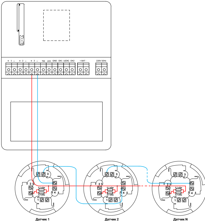
Рисунок 7. Подключение пожарных шлейфов через резисторы 5,1 кОм
