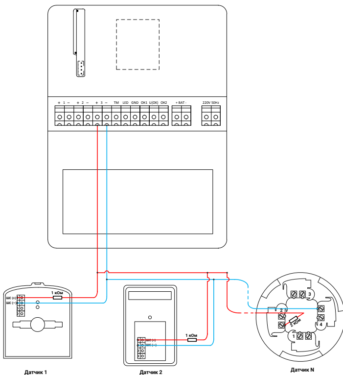
Рисунок 10. Схема подключения ручных пожарных извещателей
