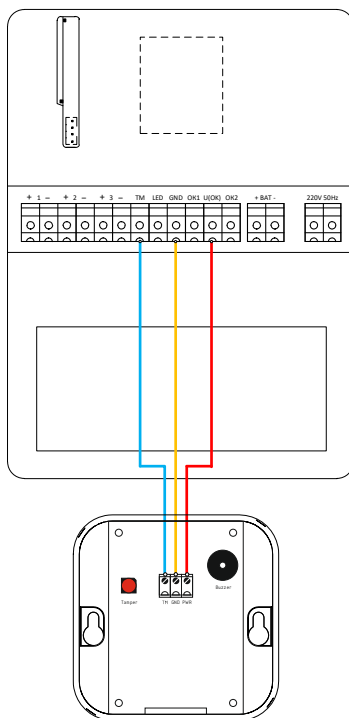
Рисунок 16. Схема подключения клавиатуры KB2-3
