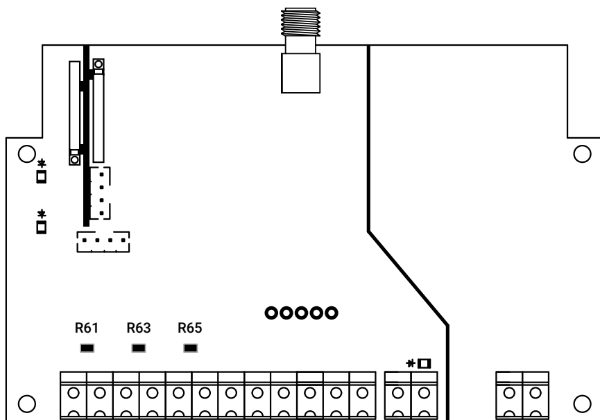
Рисунок 8. Плата панели
