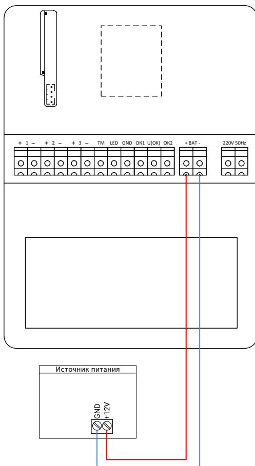
Рисунок 2. Схема подключения источника питания 12В
