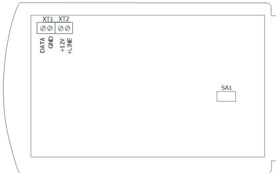
Рисунок 2. Плата клавиатуры
